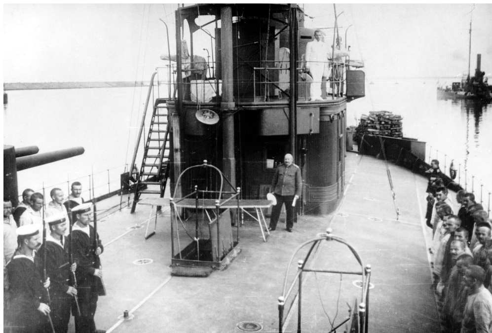
На палубе одной из башенных канонерок Амурской флотилии. Из собрания Н.Н. Афолина и архива редакции журнала «Судостроение»
